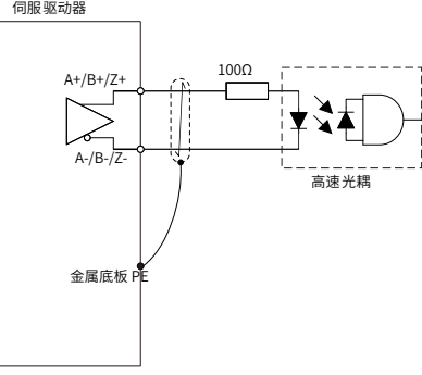
ENC2, 差分输出方式
