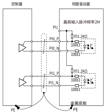
COMM1差分输入方式
