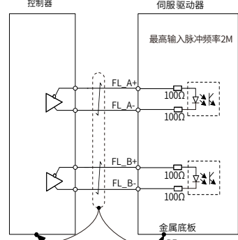
COMM2, 差分输入方式
