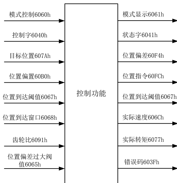
输入输出对象
