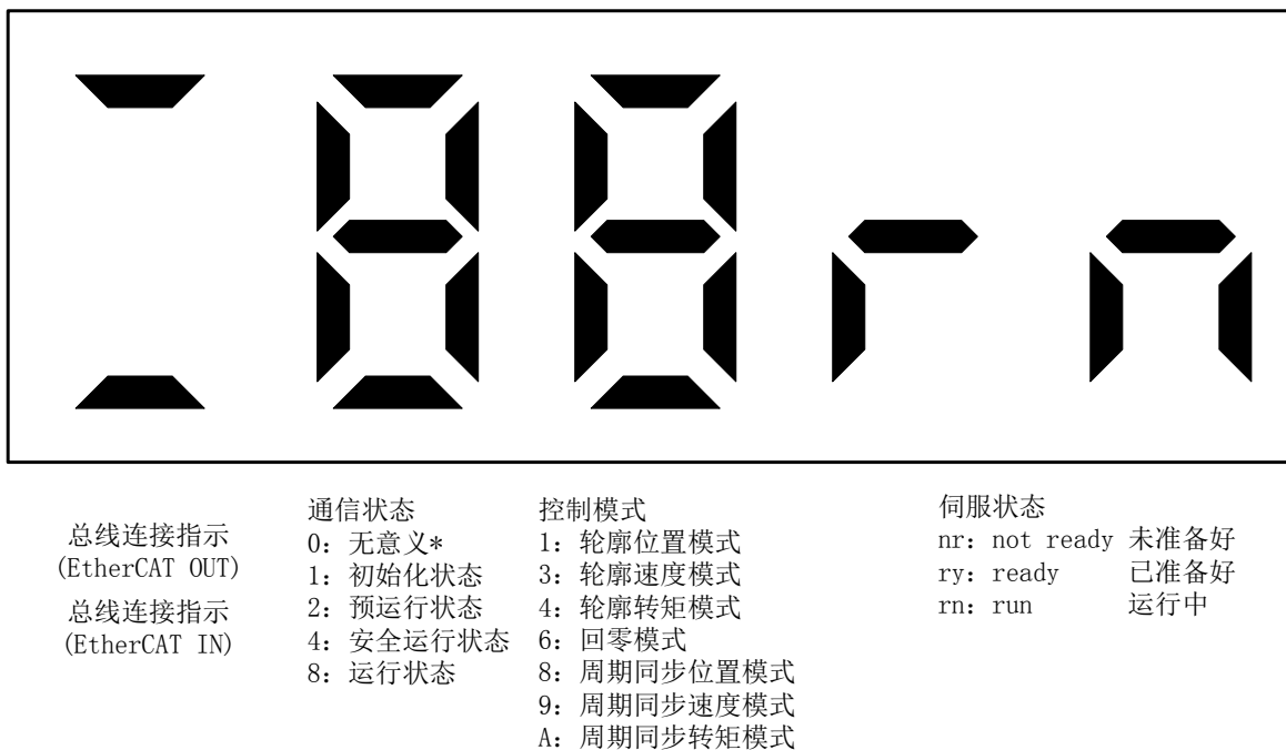
图 6-5 状态指示示意图
