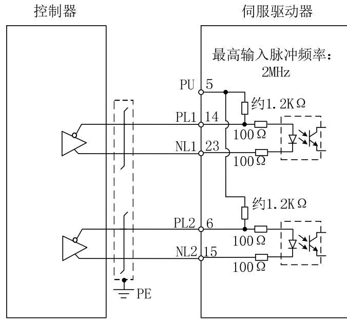
差分位置输入接线
