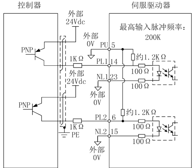
脉冲输入接线，源型方式，外部电源
