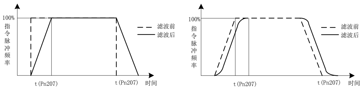
位置指令移动平均滤波器
