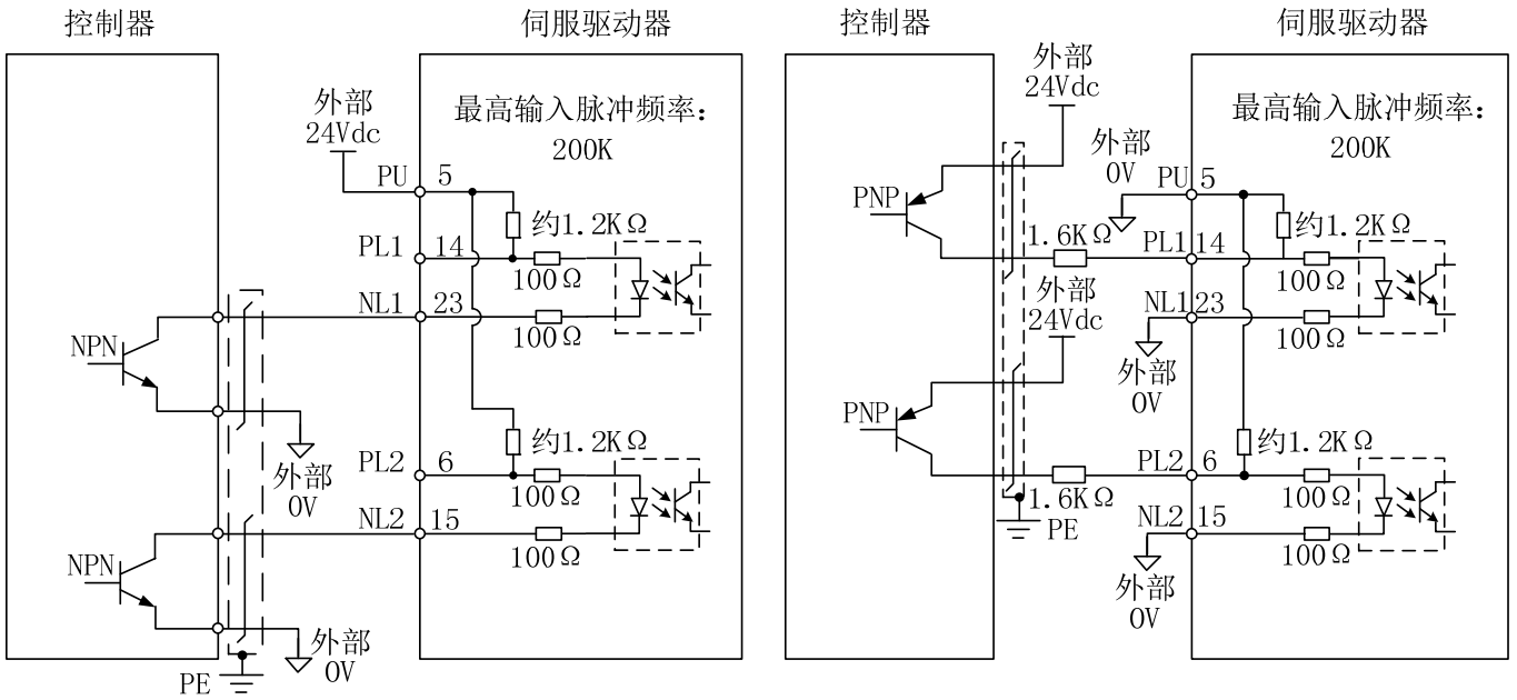
脉冲输入接线，漏型方式，外部电源
