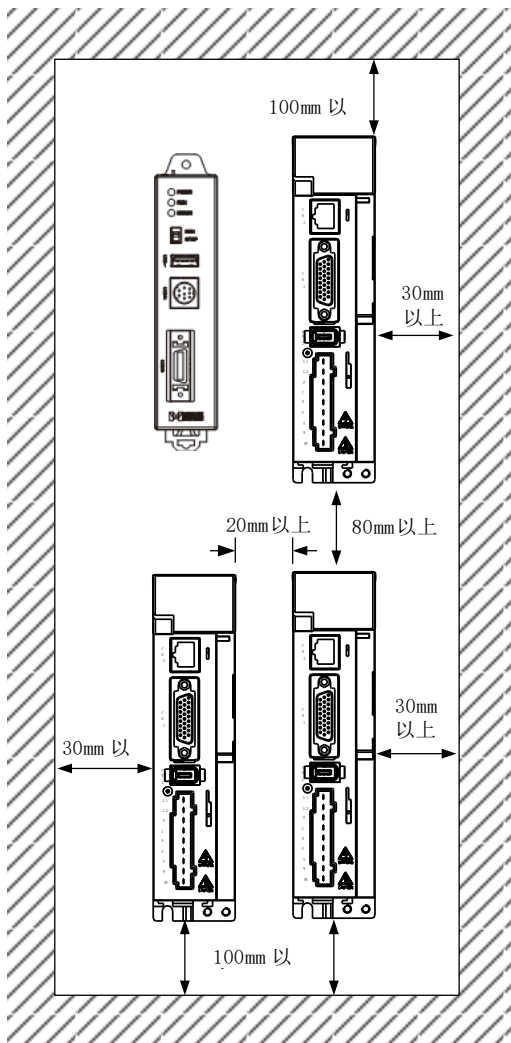
留有间隔时
