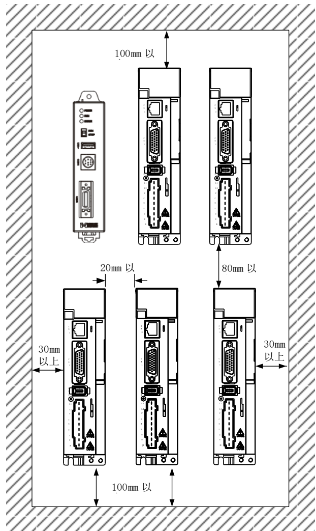
紧凑安装时
